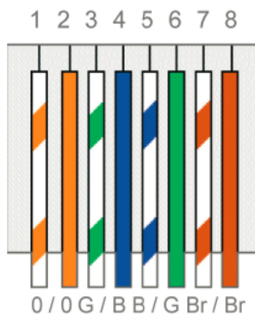
T-568B
